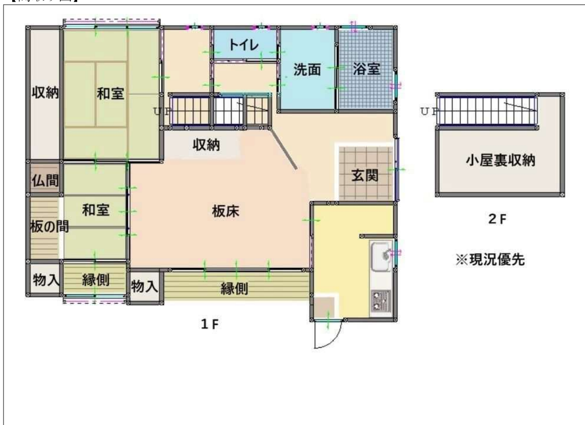
【間取り図】
