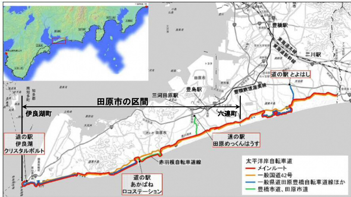
愛知県がナショナルサイクルルート指定を目指して整備する太平洋岸自転車道ルート
