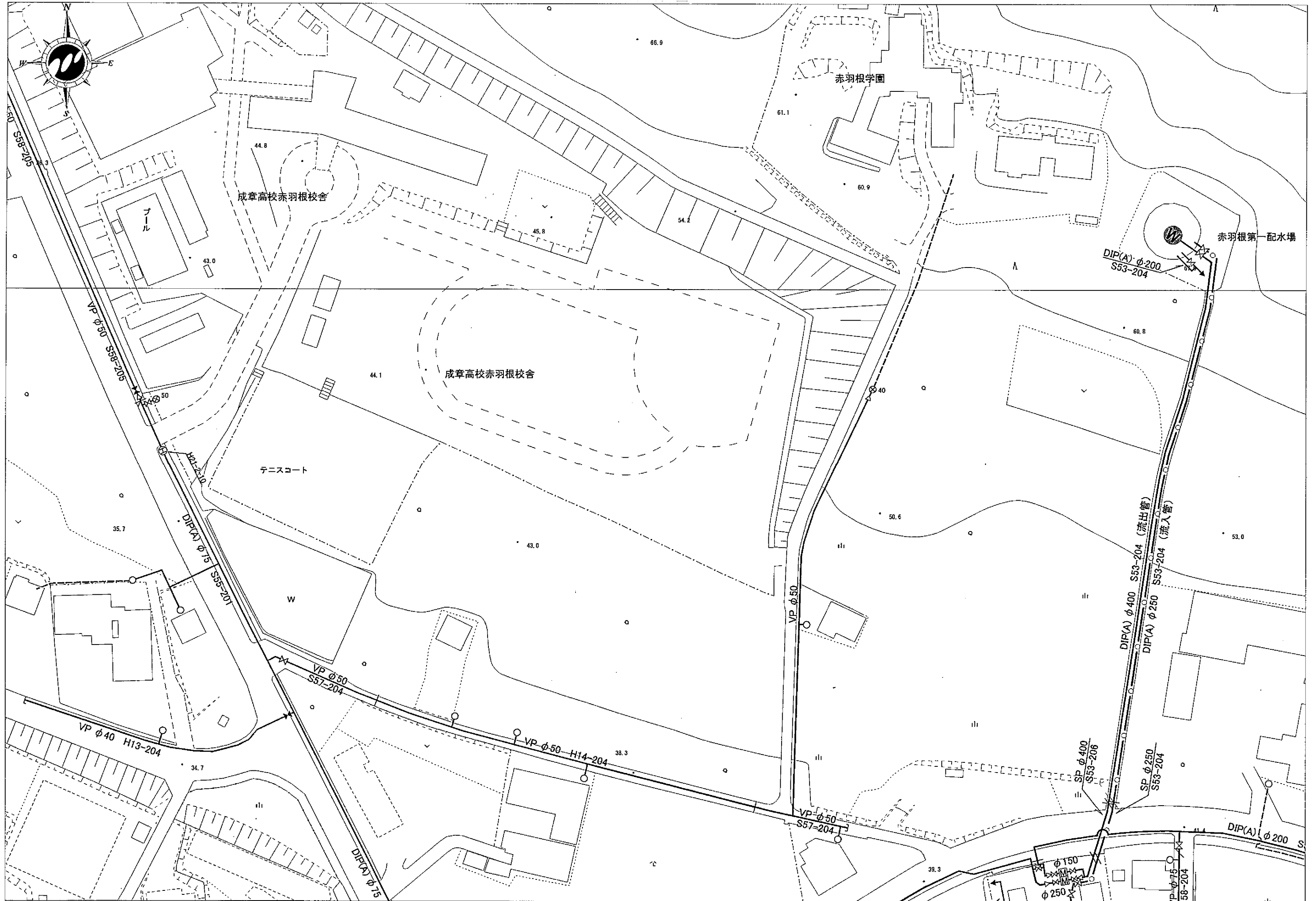
【添付資料2】上水道管理設状況図
