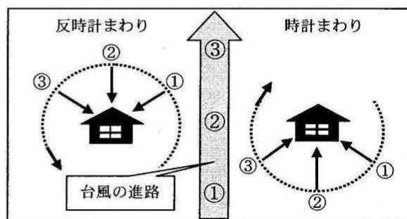
台風の進路と風向の変化
