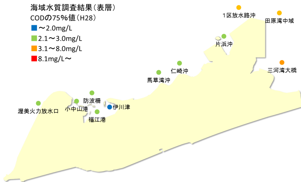
海域のCOD(H28)の75%値
