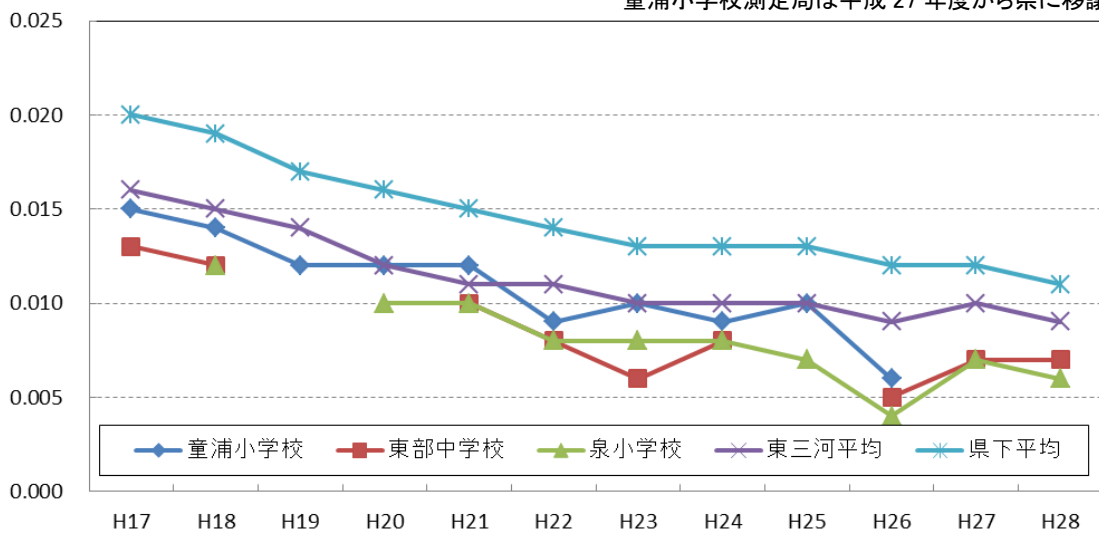
二酸化窒素の年平均値の推移
