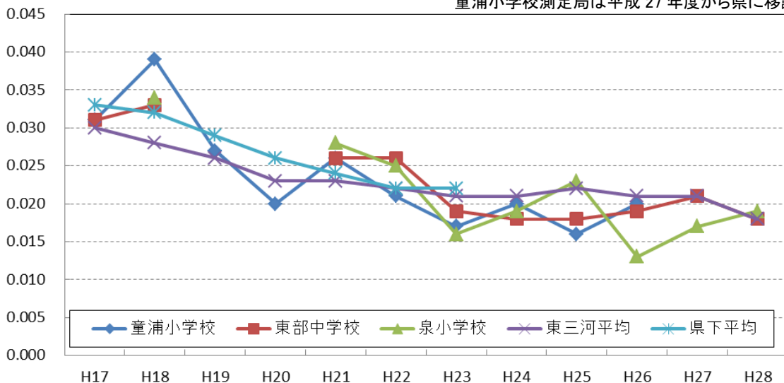
浮遊粒子状物質の年平均値の推移
