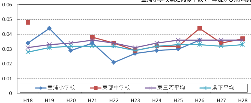
光化学オキシダントの年平均値の推移
