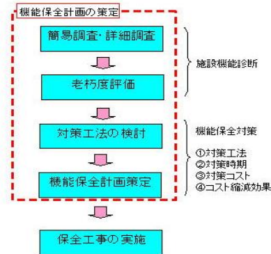
機能保全事業
